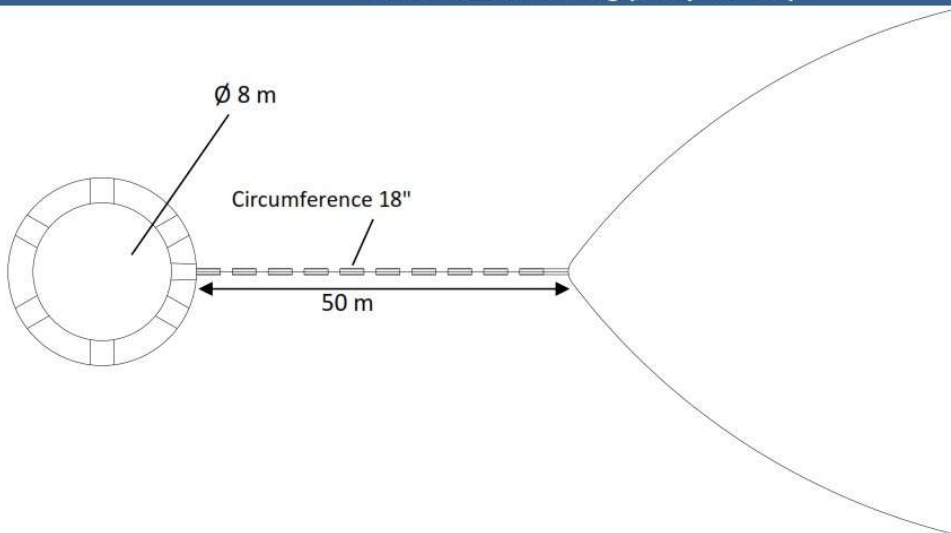
Sketsa SPM Semarang (Tampak Atas)
