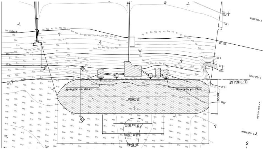
Layout TUKS Semampir Barat
